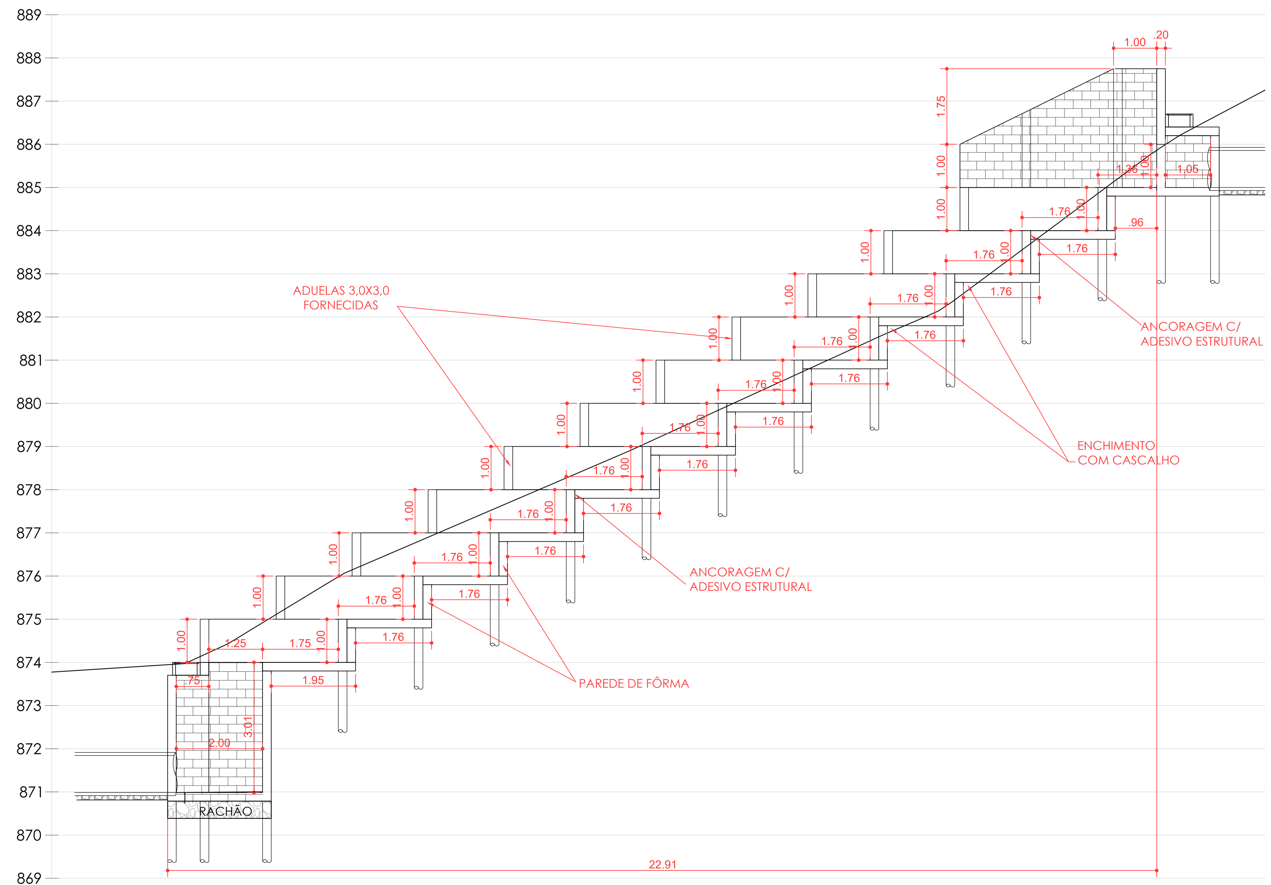
DETALHE ESCADA HIDRÁULICA - CORTE LONGITUDINAL ESC. 1:50
