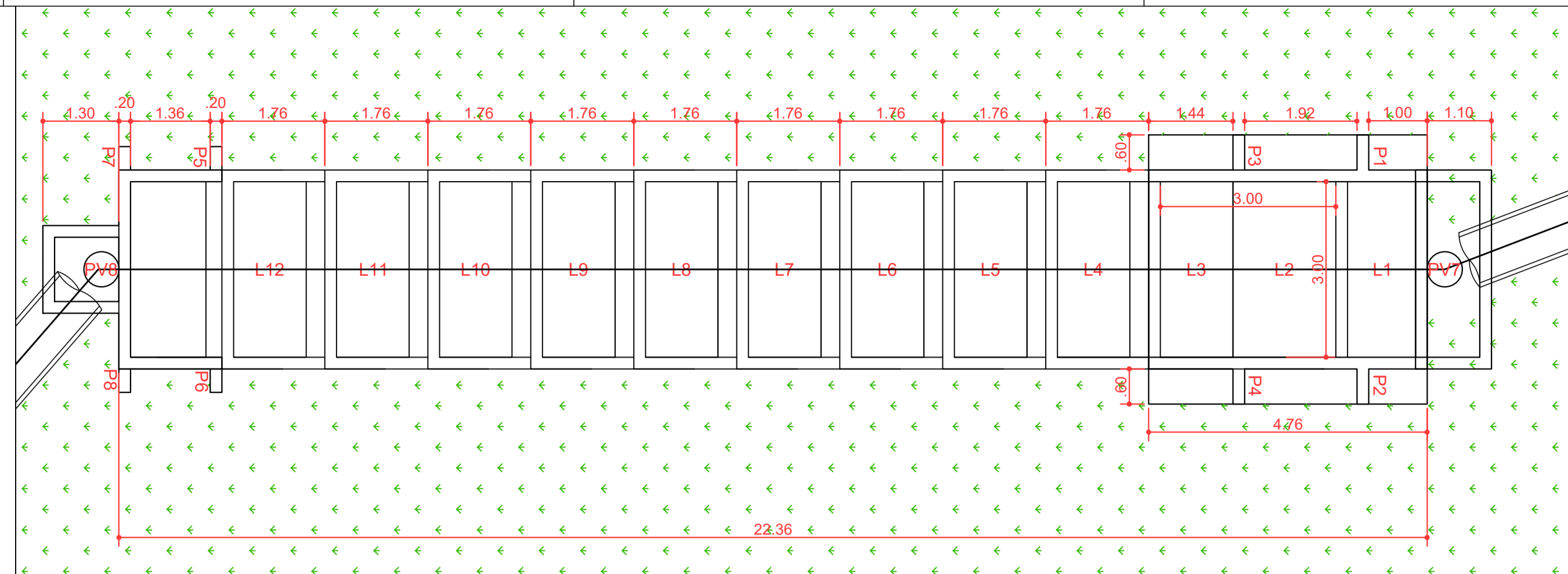
DETALHE ESCADA HIDRÁULICA - PLANTA ESC. 1:75
