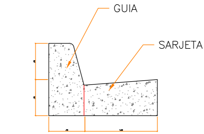
DETALHE GUIA E SARJETA S/ESCALA
