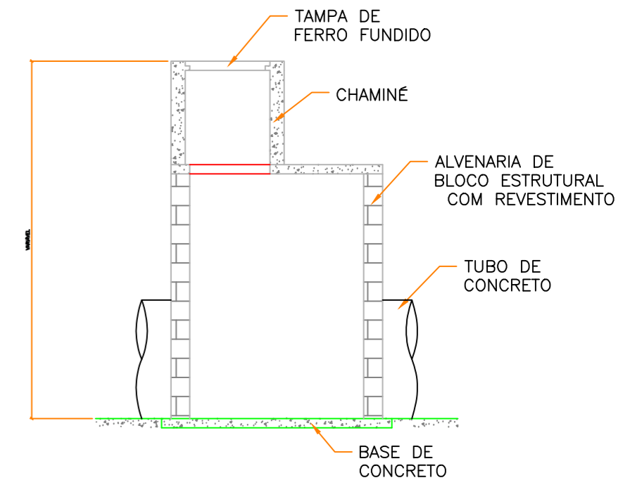
SEÇÃO TRANSVERSAL POÇO DE VISITA S/ESCALA
