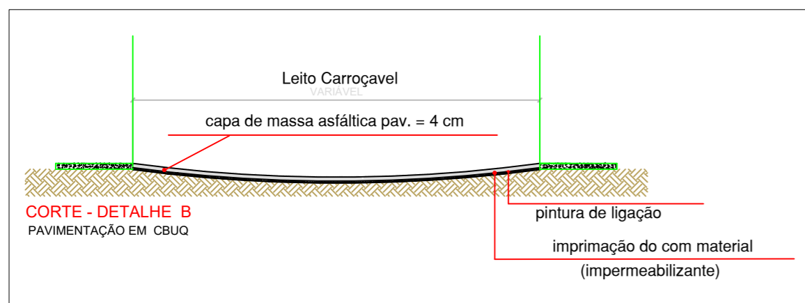
SEÇÃO TRANSVERSAL DO PAVIMENTO - PAVIMENTAÇÃO DA VIELA S/ESCALA
