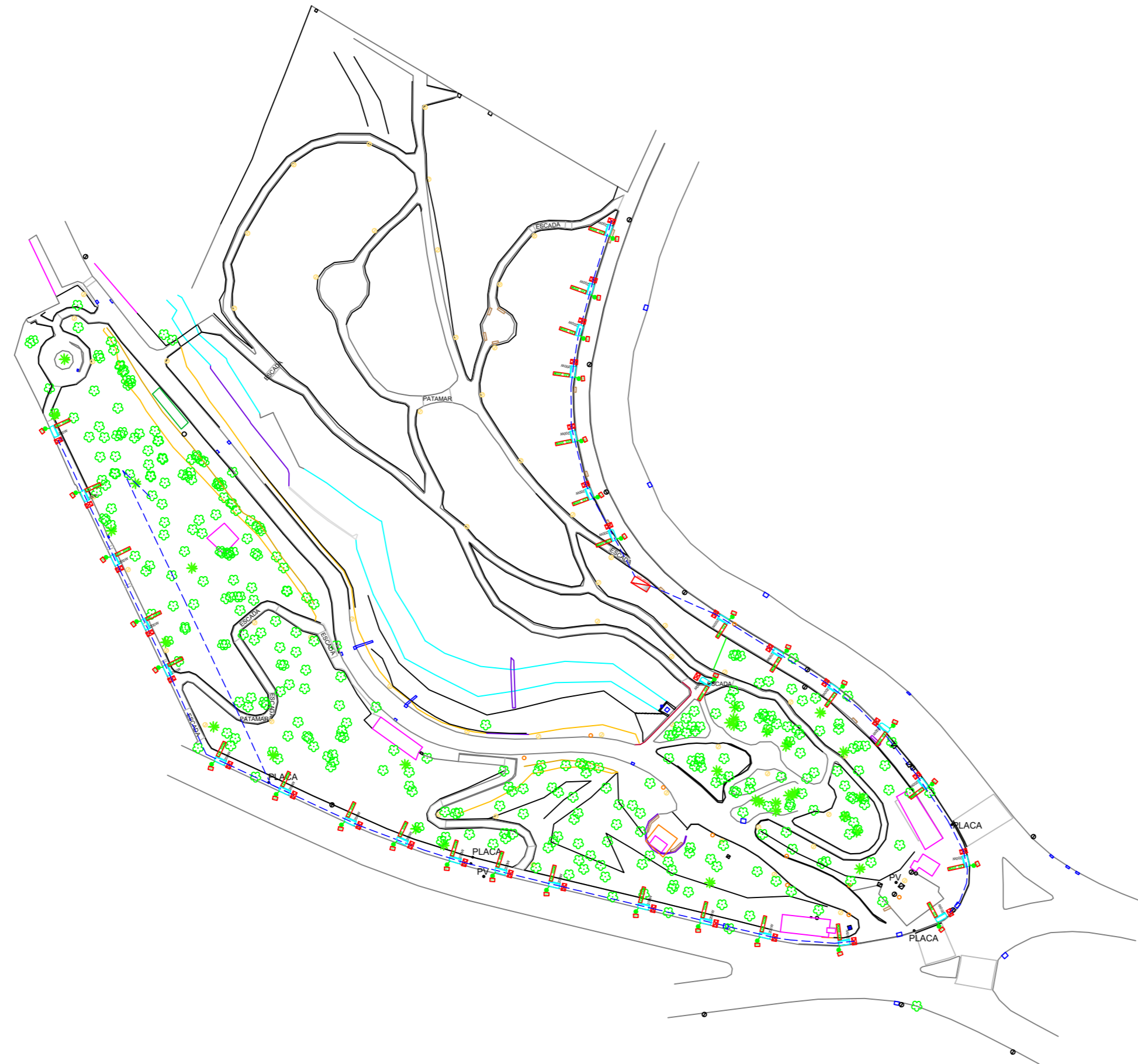
BOSQUE ZEQUINHA DE ABREU - ILUMINAÇÃO PROJETADA ESCALA 1: 1000
